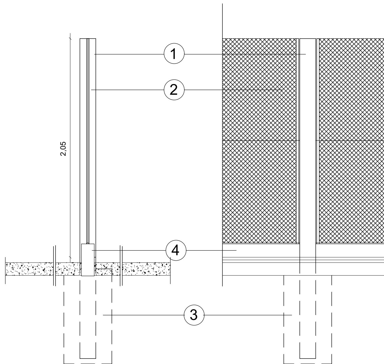
CORTE TRANSV.
