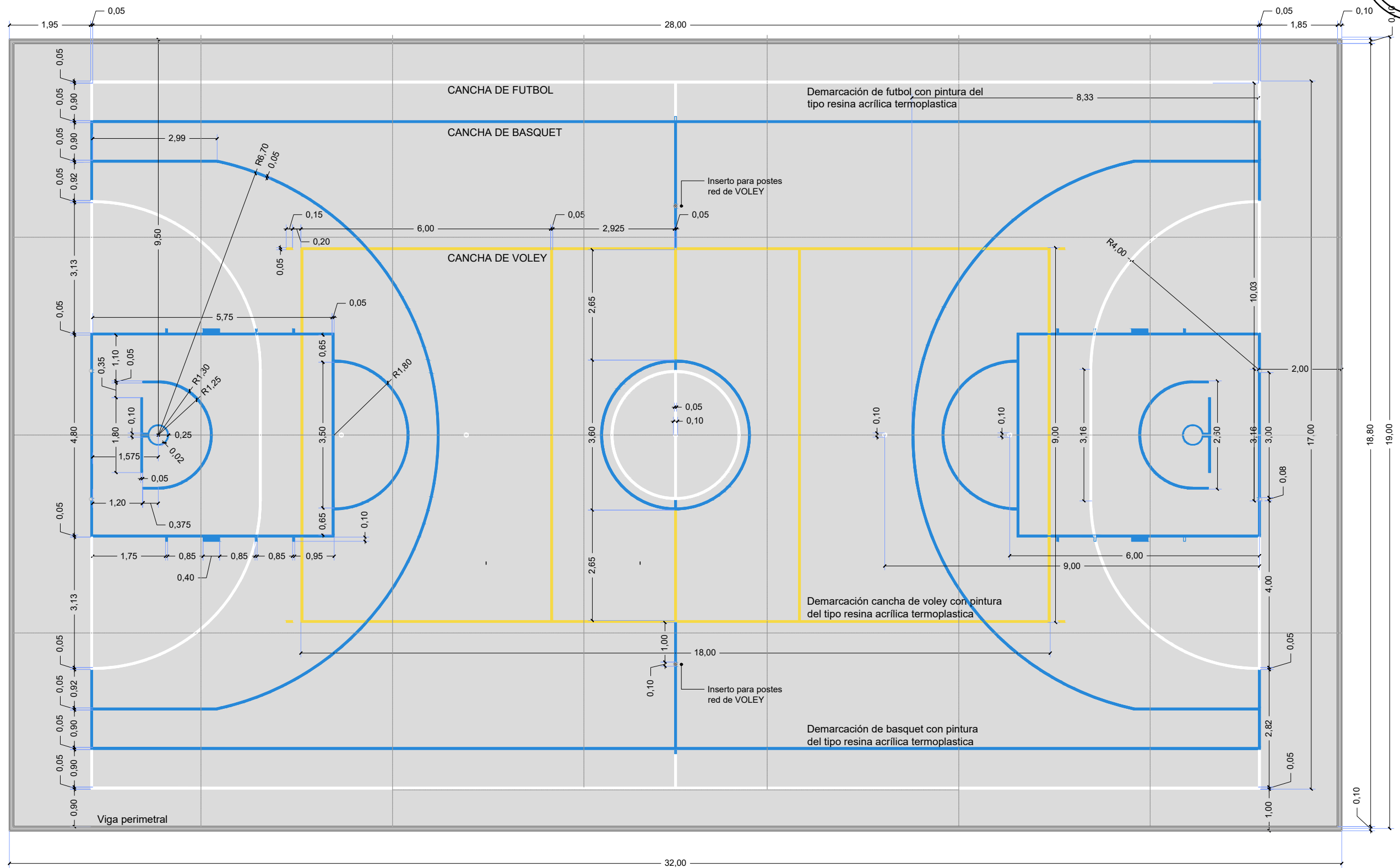
PLAYON DEPORTIVO CANCHAS DE BASQUET, FUTBOL DE SALON Y VOLEY ESQUEMA DE MARCADO Esc. 1:100
